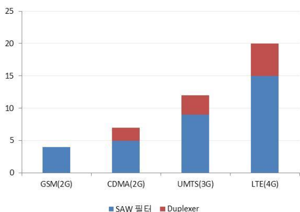
그림 14. SAW 필터/듀플렉서 사용량 (단위: 개)
