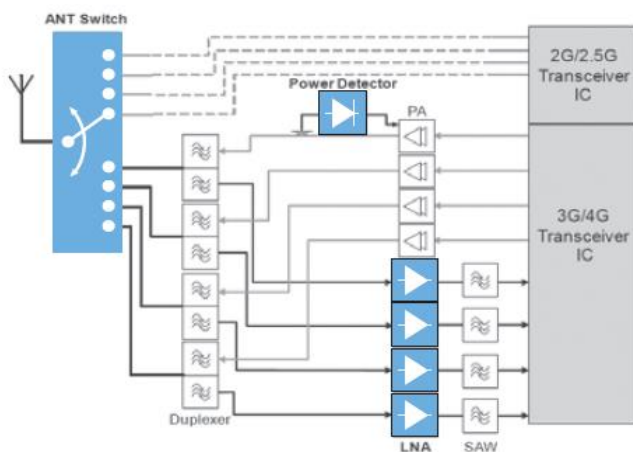
그림 1. 스마트폰의 메인 Cellular RF 다이어그램
